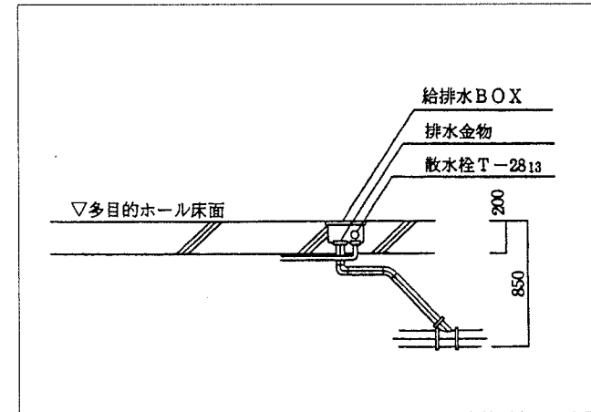
多目的ホール内給排水ボックス詳細図
